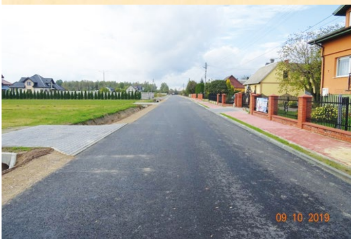
z Funduszu Dróg Samorządowych w łącznej kwocie: 1.185.888 zł. Przebudowa drogi dojazdowej do pól uprawnych w Grzybowej Górze na działce nr 14 - etap II objęła wykonanie odcinka dł. 95,00 m, podbudowy z kruszywa łamanego, pobocza z zamknięciem
